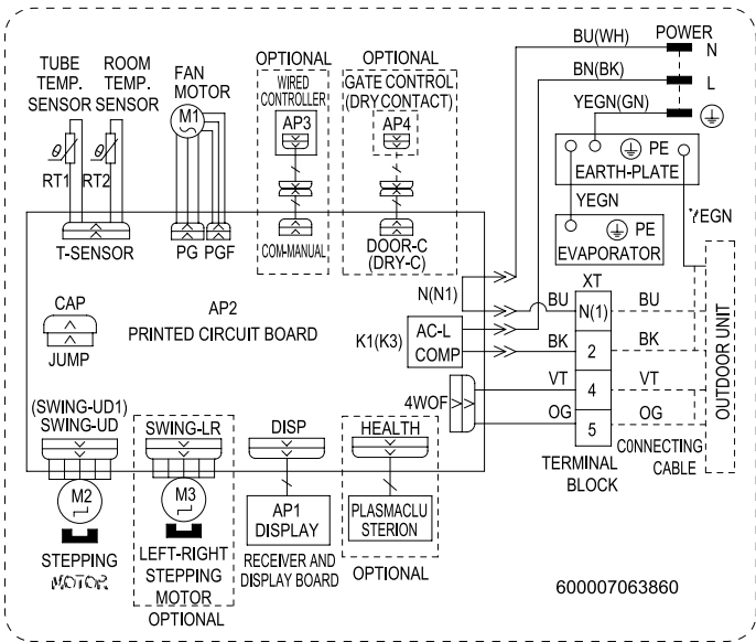
Внутренний блок KVAC-18IN-FP1, KVAC-24IN-FP1
