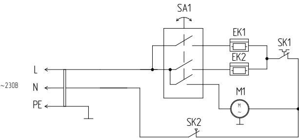
Схема коммутации переключателя
