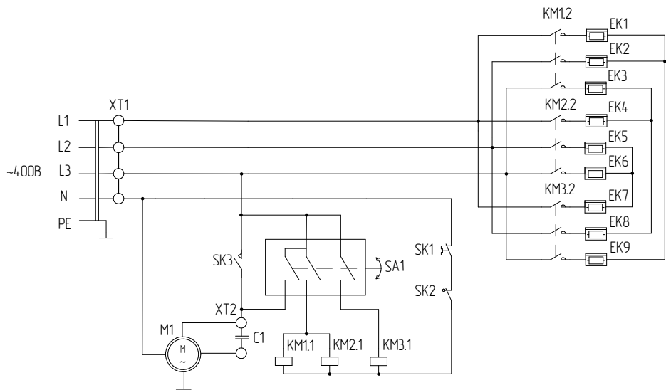
Схема коммутации переключателя
