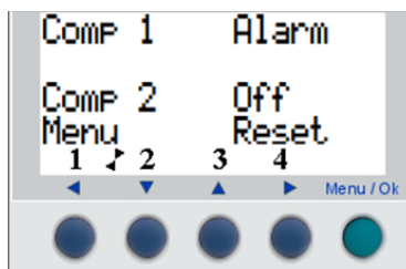
Рисунок 1. Компрессор 1 – авария, Компрессор 2 – выключен.
